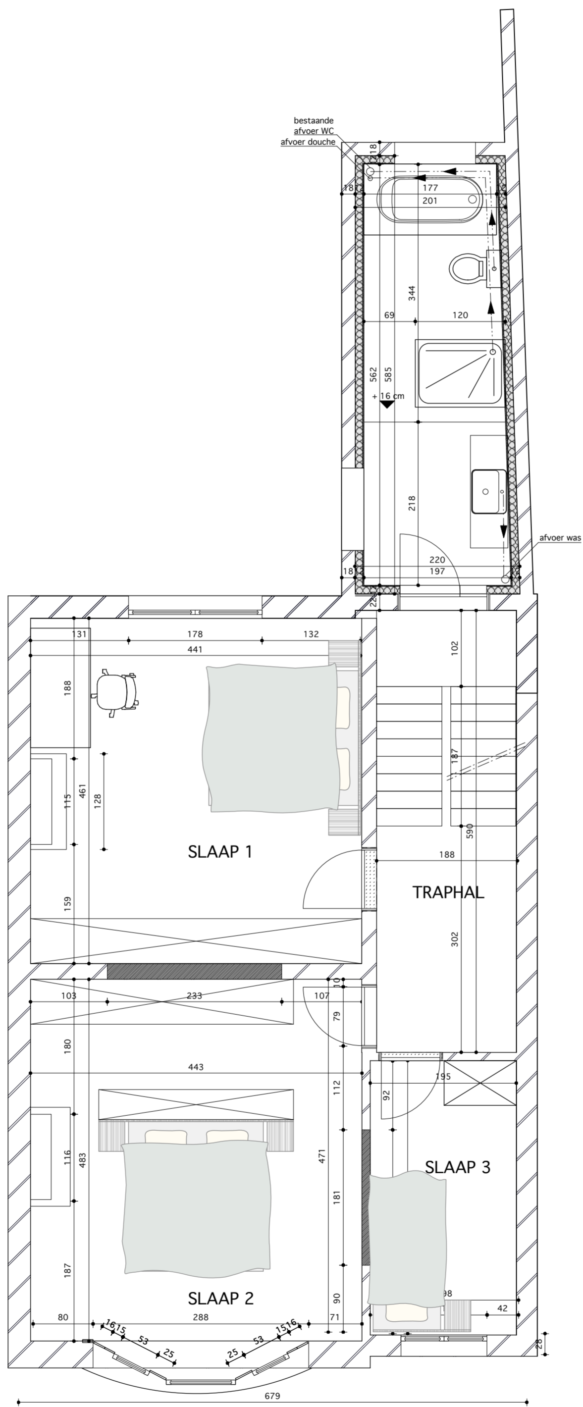
VERDIEPING nieuwe toestand- voorstel 1 schaal 1/50
